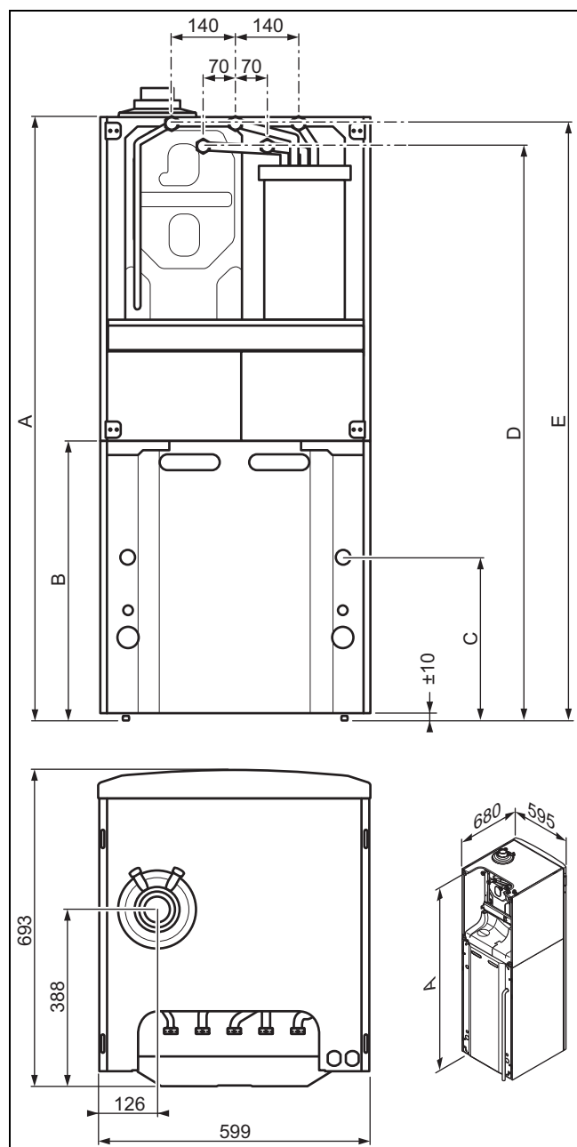
Rozměry zařízení
